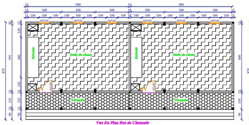
Plan de construction d'un bloc de 2 classes
