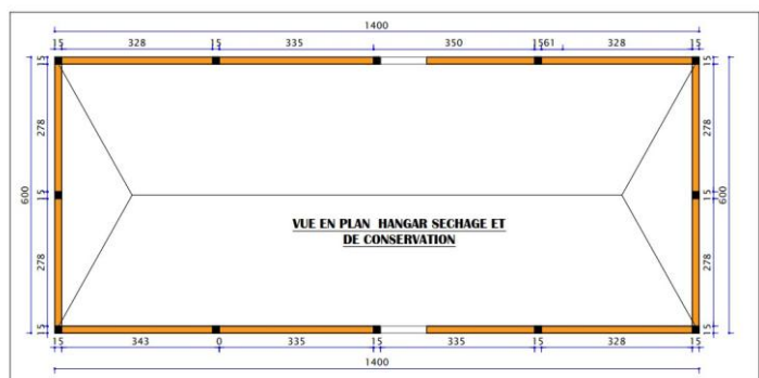
Maquette et plan du hangar de séchage et de conservation
